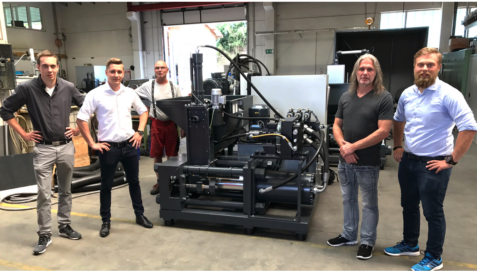
FAT-test utförs på den kundanpassade brikettpressen hos Weima. Till vänster om pressen ses personal från Weima, sedan Peter Torvaldsson, Ljunghäll och längst till höger Patrick Hörmann, projektledare Mercatus.
